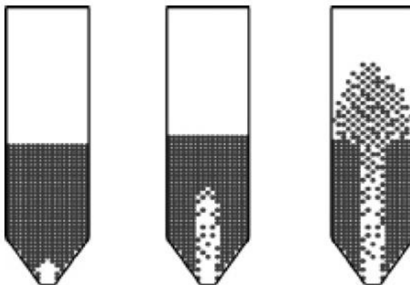
Figura 1- Esquema de evolução do processo de jorro.
