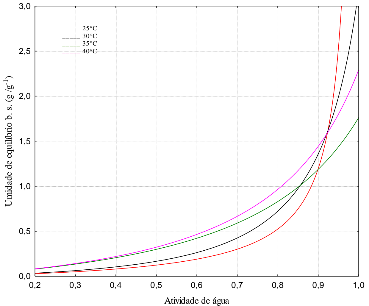
Figura 17 – Isotermas de adsorção do suco de caju em pó nas temperaturas experimentais de 25, 30, 35 e 40°C (linhas) prevista pelo modelo de BET.
