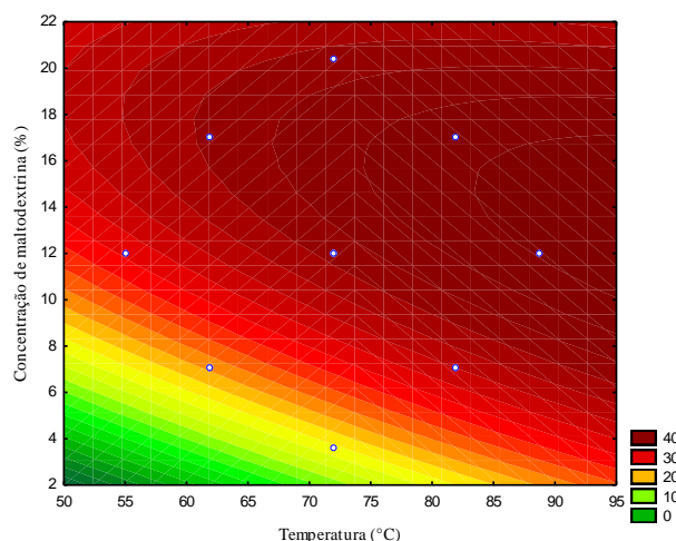
Figura 12 – Curva de contorno concentração de maltodextrina versus a temperatura para variável resposta rendimento.
