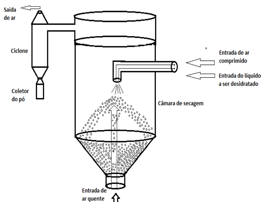
Figura 2 - Esquema de um secador leito de jorro com partículas inertes.
