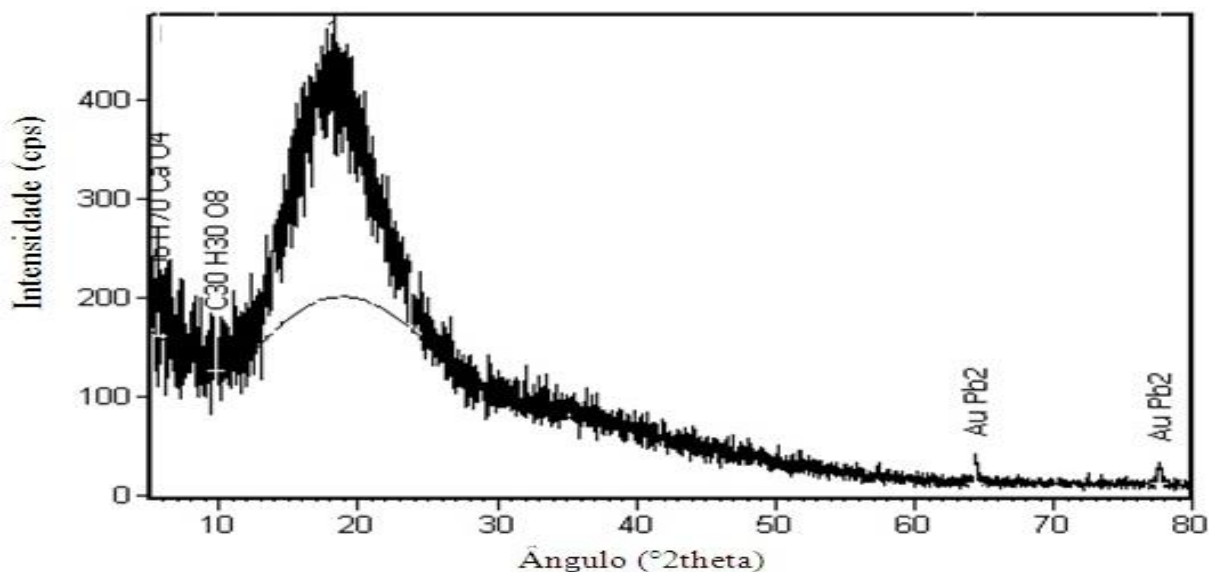
Figura 13 – Difratoograma do suco de caju em pó obtido em leite de jorro.
