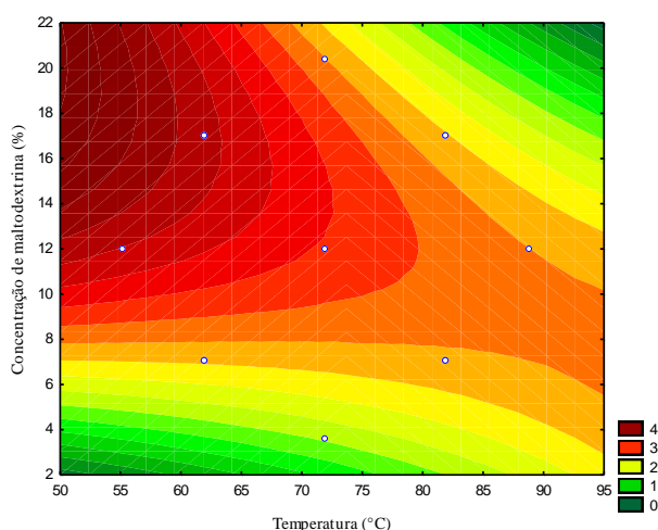
Figure 9 - Curva de contorno concentração de maltodextrina versus a temperatura para a variável resposta umidade
