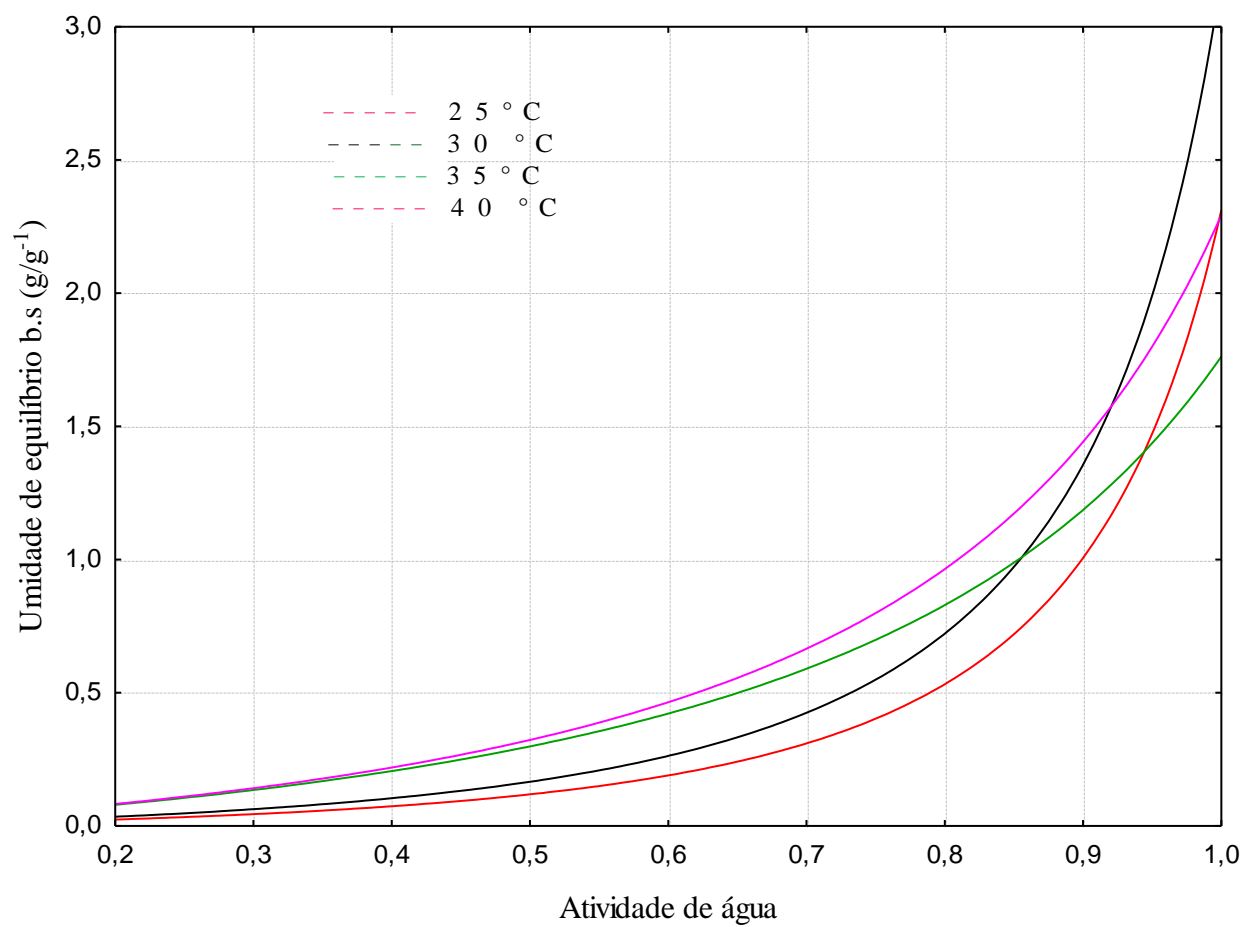
Figura 18 – Isotermas de adsorção do suco de caju em pó nas temperaturas experimentais de 25, 30, 35 e 40°C (linhas) prevista pelo modelo de GAB.
